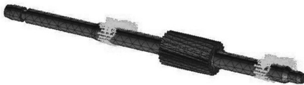
Рис. 2. Конечно-элементная модель приводного вала
