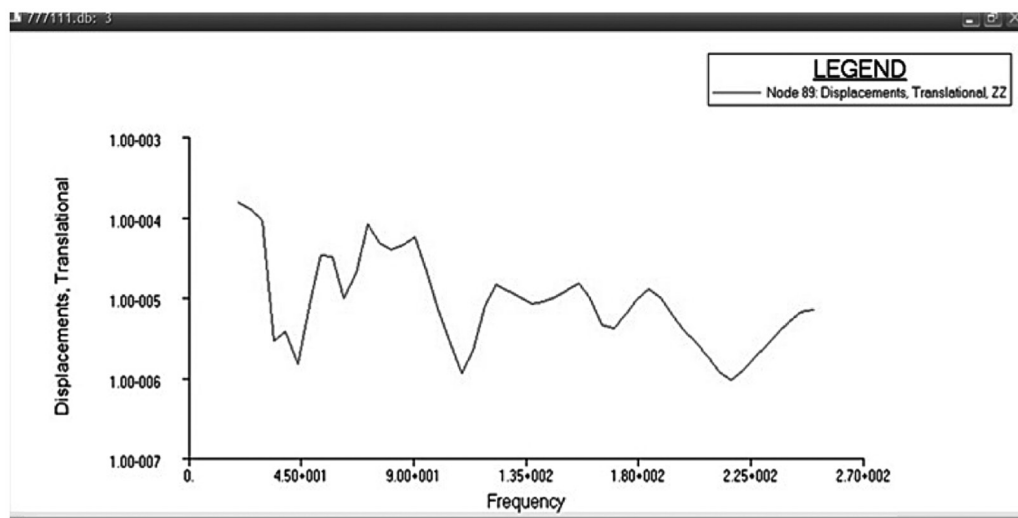
Рис. 5. Амплитудно-частотная характеристика
