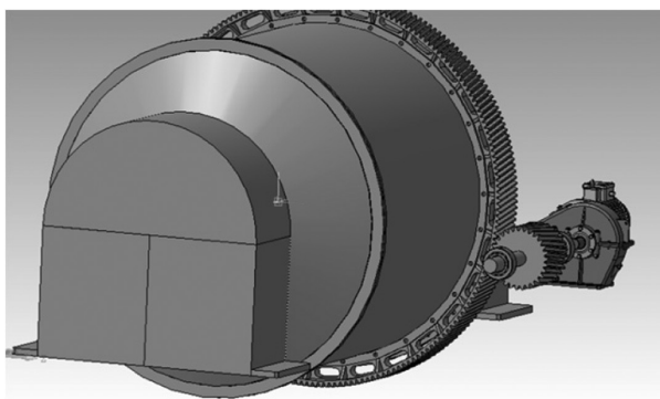
Рис. 1. 3D модель системы привода шаровой мельницы
